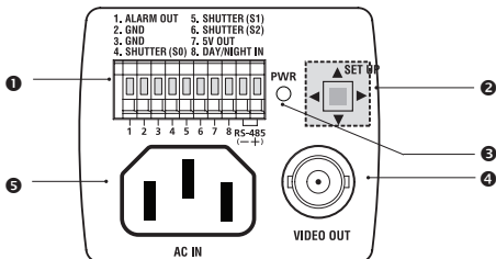
<AC220V~240V(SCB-2001PH)>
