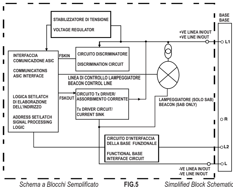
Schema a Blocchi Semplificato
