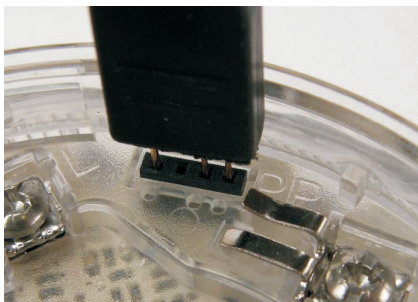
Fig. 4 FC490ST Programming Lead and FC430LP Programming Port Interface. Connettore di Programmazione del FC490ST e Porta di Programmazione del FC430LP.
