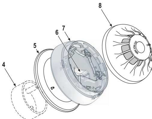
Fig. 2 Einbau des FC-Meldersockels mit dem Aufputzsocket Typ A. Fitting to a flat surface. Montaggio su una superficie piana.
