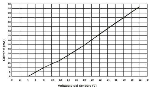
Fig. 3 Grafico Corrente di allarme/Tensione sensore
