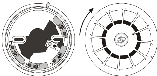
Fig. 4 Montaggio del sensore 601H-R / 601H-F sulla base MUB: 1- posizionare il sensore sopra la base nella posizione relativa indicata in figura; 2- ruotare il sensore sulla base nel senso della freccia fino al bloccaggio.
