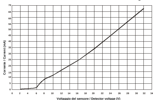
Fig. 3 Grafico Corrente di allarme/Tensione sensore / Alarm load
