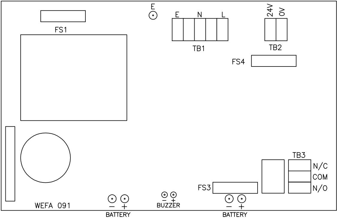
27.6V 1A MONITORED LINEAR CHARGER
